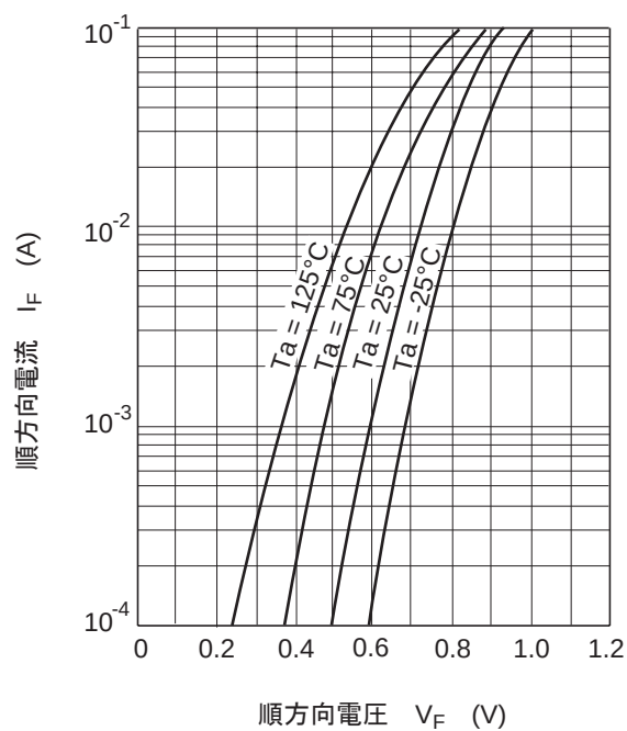
図1. 順方向特性
