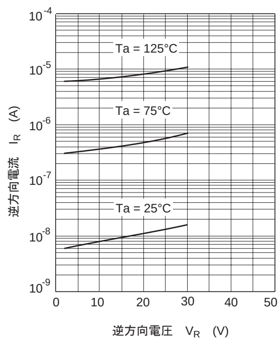
図2. 逆方向特性
